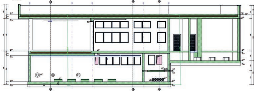
Pumpstation und Beschneigungsleitung | Mühlbach am Hochkönig
