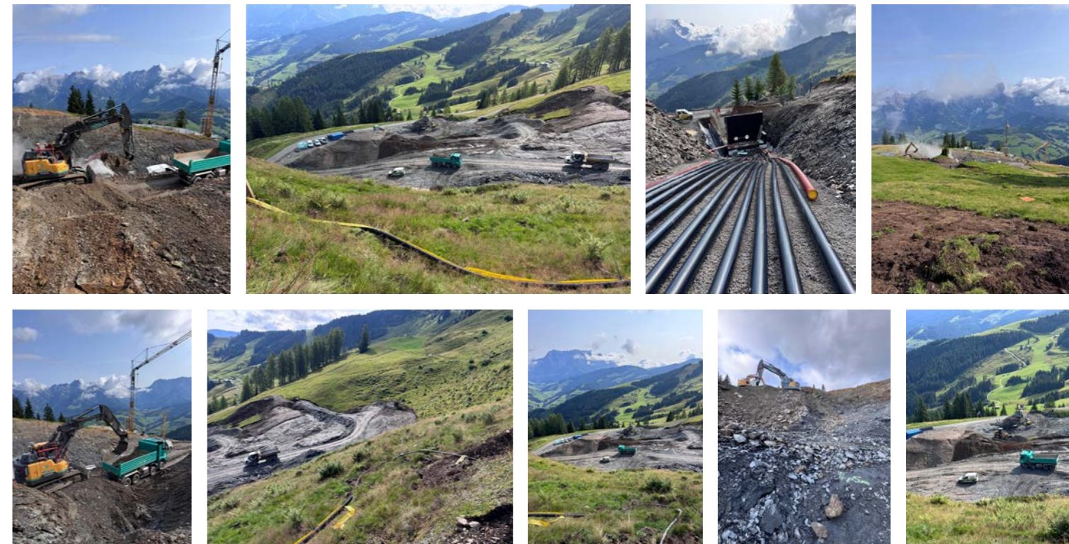
Hoch- und Tiefbau Abergbahn | Hochkönig
