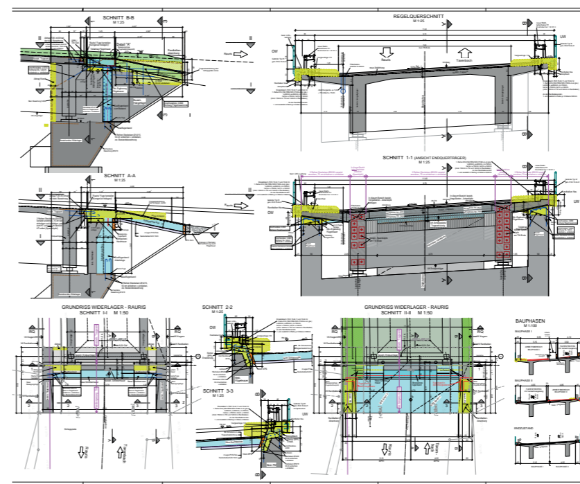
Generalsanierung Trieglergrabenbrücke | Rauris
