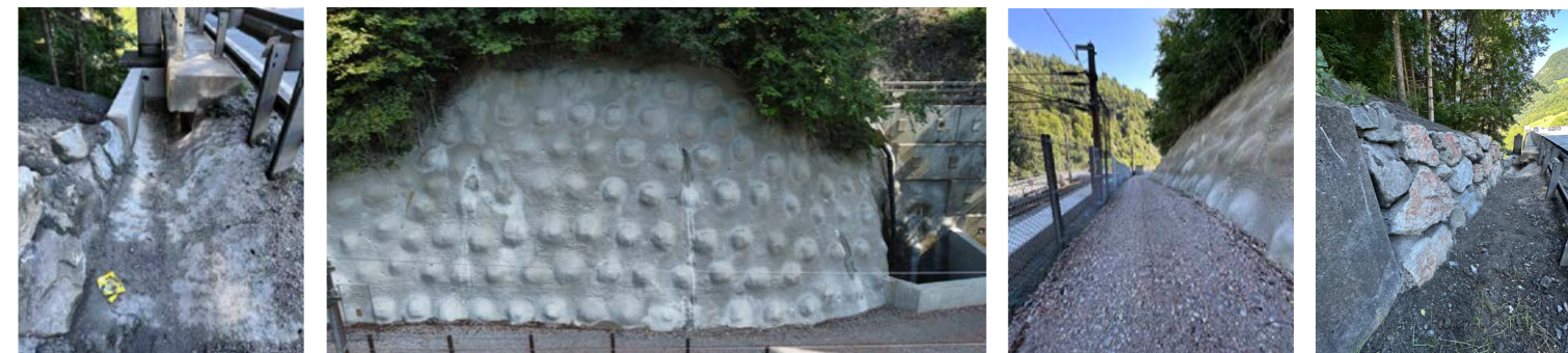
B311 Entwässerungssanierung | Lend
