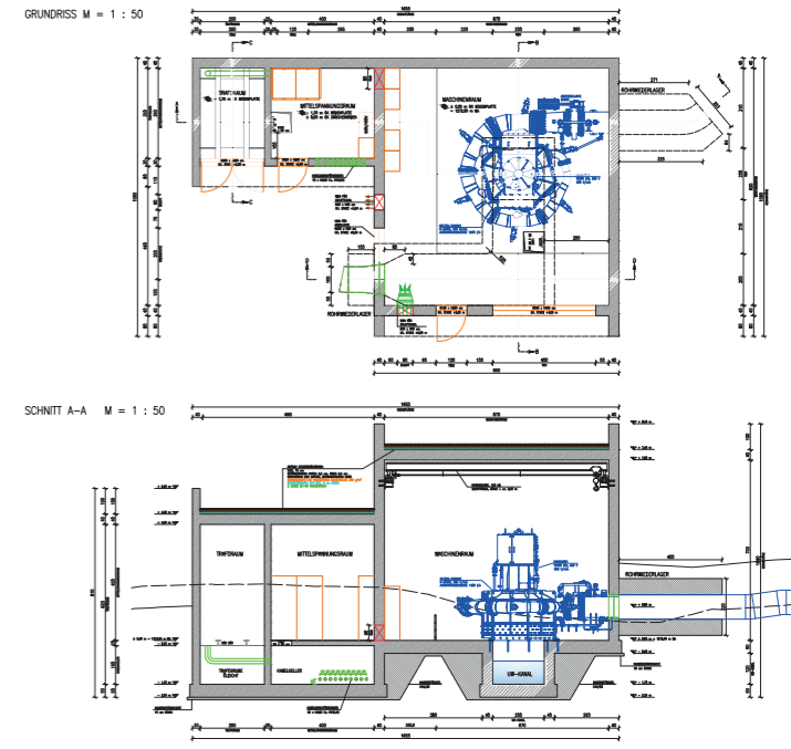
Wasserkraftwerk Krumbach - Wasserrfassung, Druckrohrleitung und Krafthaus | Gerlos
